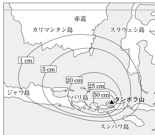
図 5 1815 年に起こったタンボラ山の噴火による降灰分布
