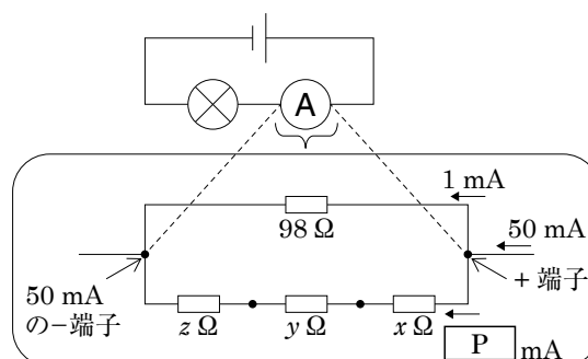
図 9 50 mA の－端子につないだとき
