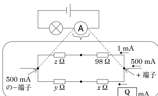
図 10 500 mA の－端子につないだとき
