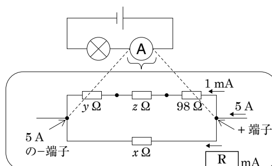
図 11 5 A の－端子につないだとき
